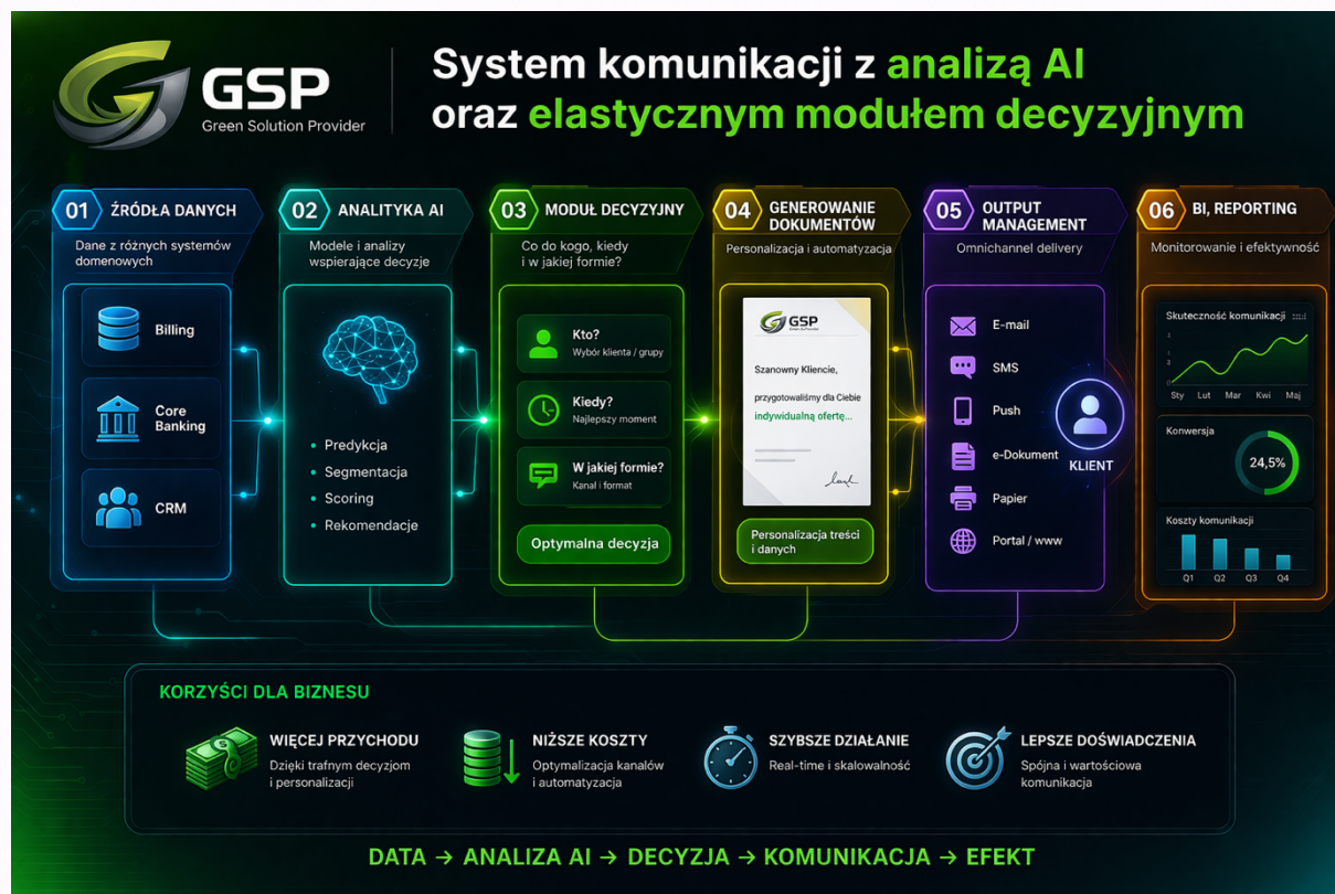
Rys. 1 GSP Suite
